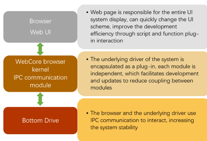
Web UI Frame
